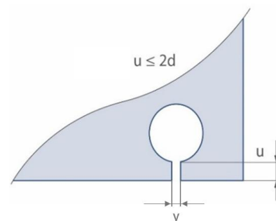
Fig. 14 Relief cut
